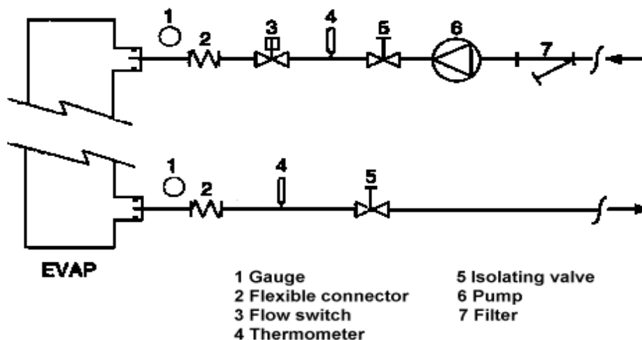
Fig. 6 - Conexión de tuberías de agua para evaporador
