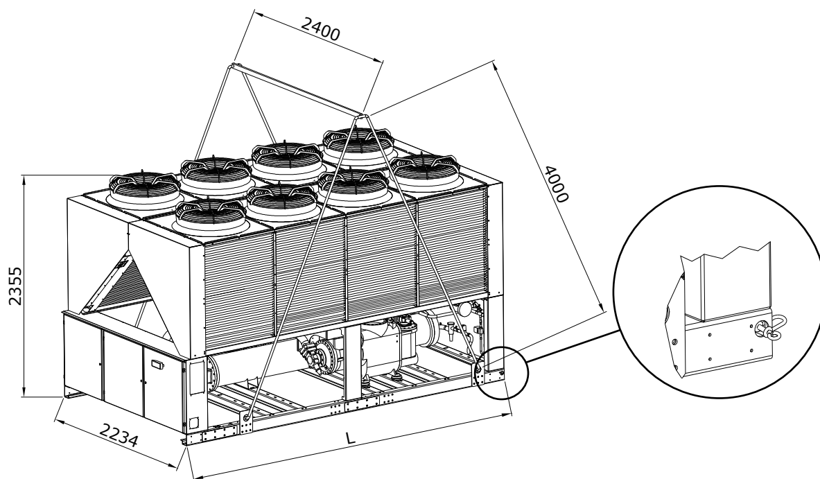
Fig. 3 – Izado de la unidad
