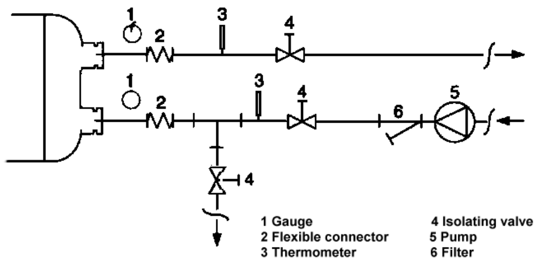
Fig. 7 - Conexión de tuberías de agua de los intercambiadores de recuperación de calor
