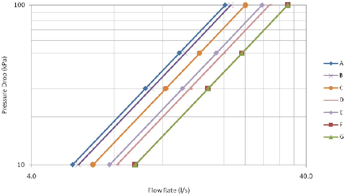
Fig. 12 – Caída de presión a través del evaporador
