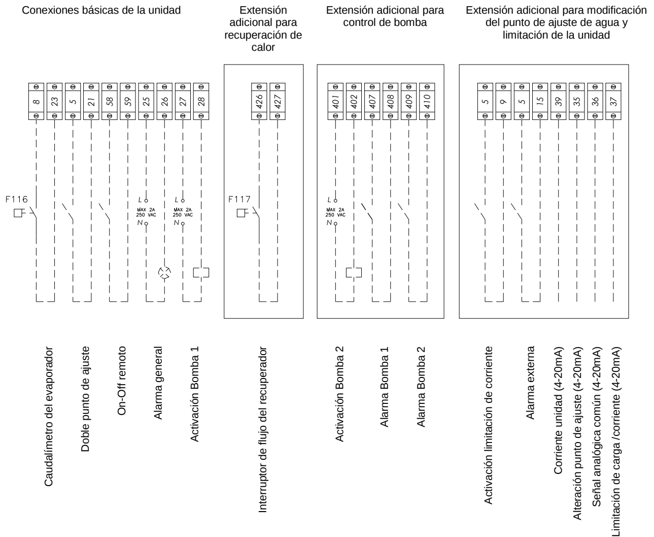
Fig. 14 – Conexiones de usuario al panel interfaz de terminales M3
