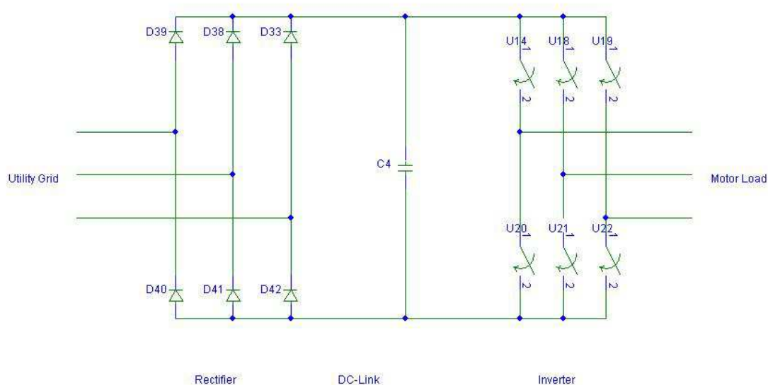
Fig. 16 – Diagrama típico de un VFD
