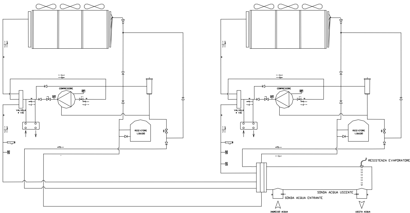
Fig. 21 – Ciclo frigorífico con recupero di calore parcial
