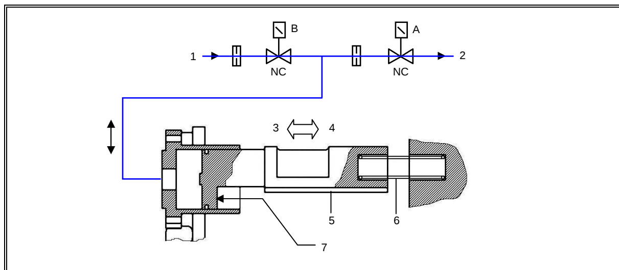
Fig. 24 – Mecanismo de control de capacidad del compresor Fr3100
