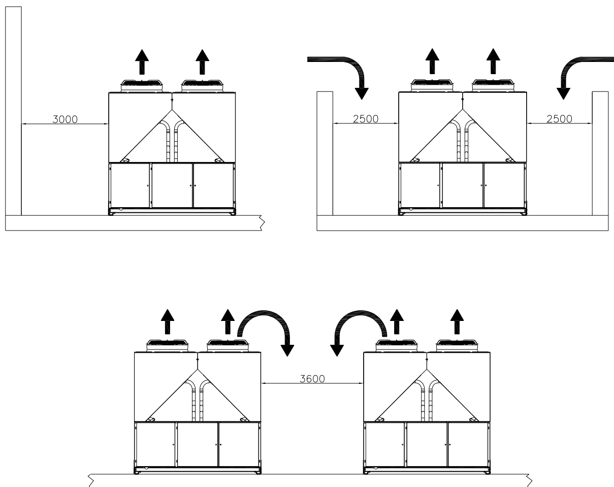
Fig. 5 – Distancias mínimas de instalación recomendadas
