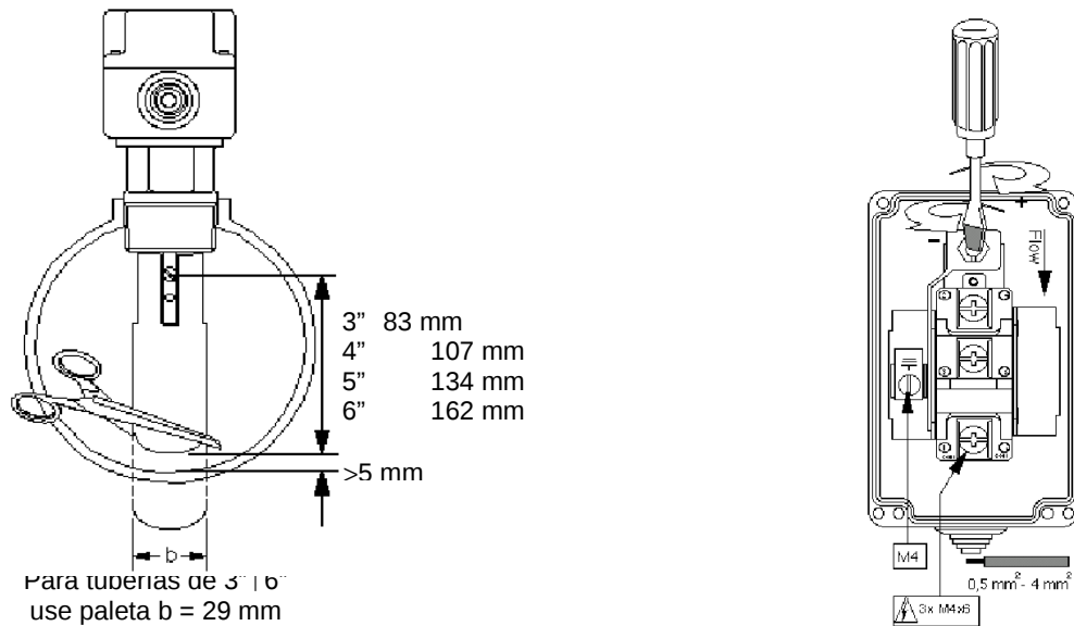
Fig. 8 – Ajuste del interruptor de flujo
