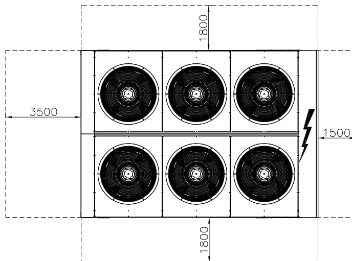
Fig. 4 – Requisitos mínimos de espacio para mantenimiento de la unidad
