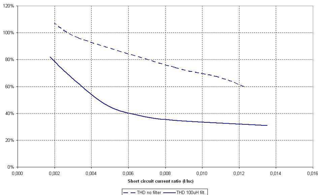
Fig. 18 – Contenido armónico con o sin inductancia de línea
