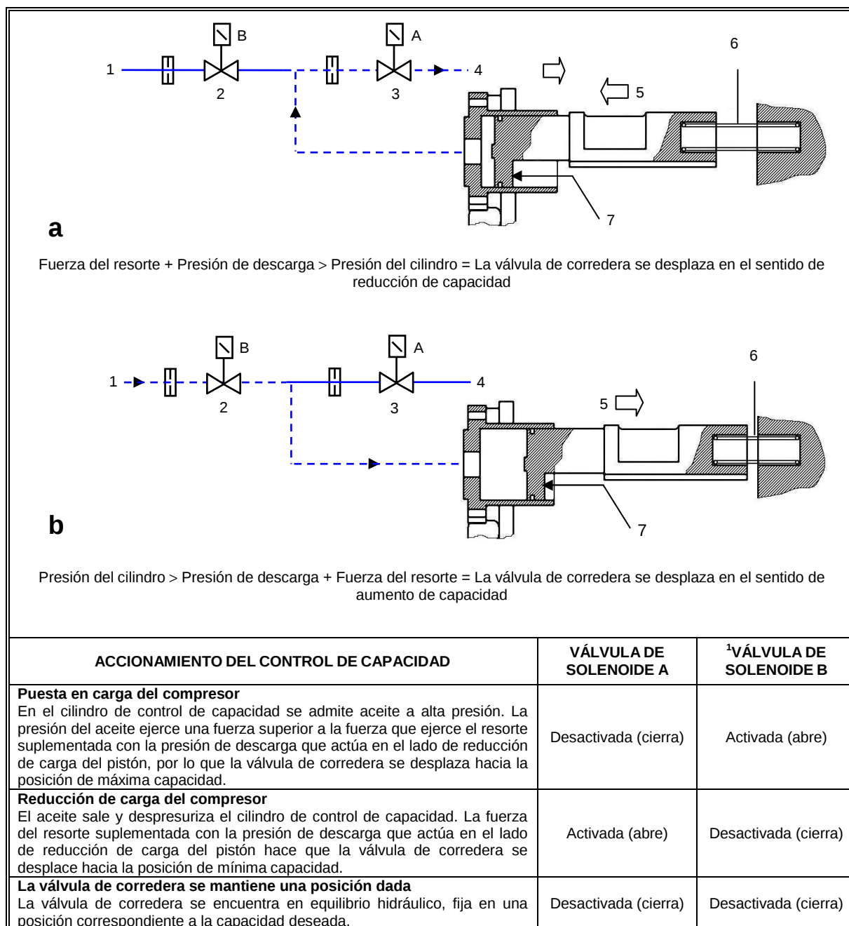
Fig. 25 – Control progresivo de capacidad del compresor Fr3100
