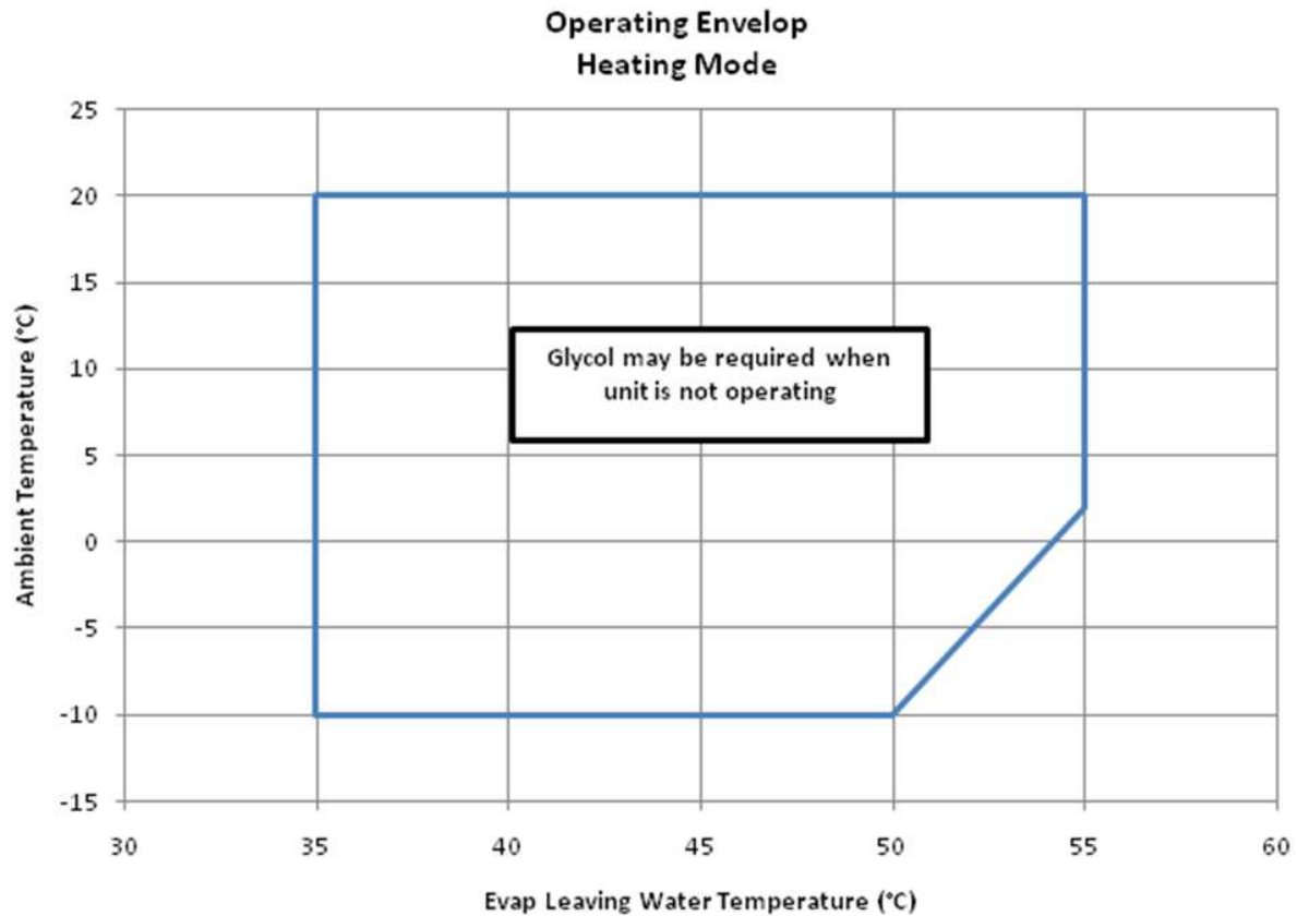
Fig. 2 – Limites Operativos en calor – EWYD-BZSS / EWYD~BZSL
