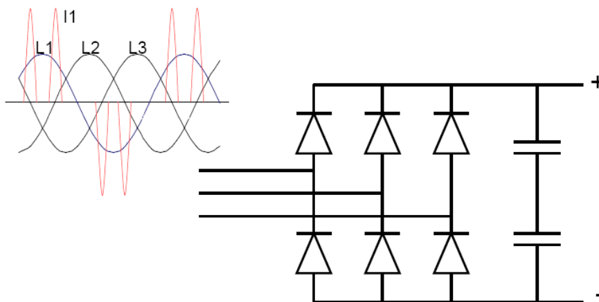
Fig. 17 – Armónicas en la red
