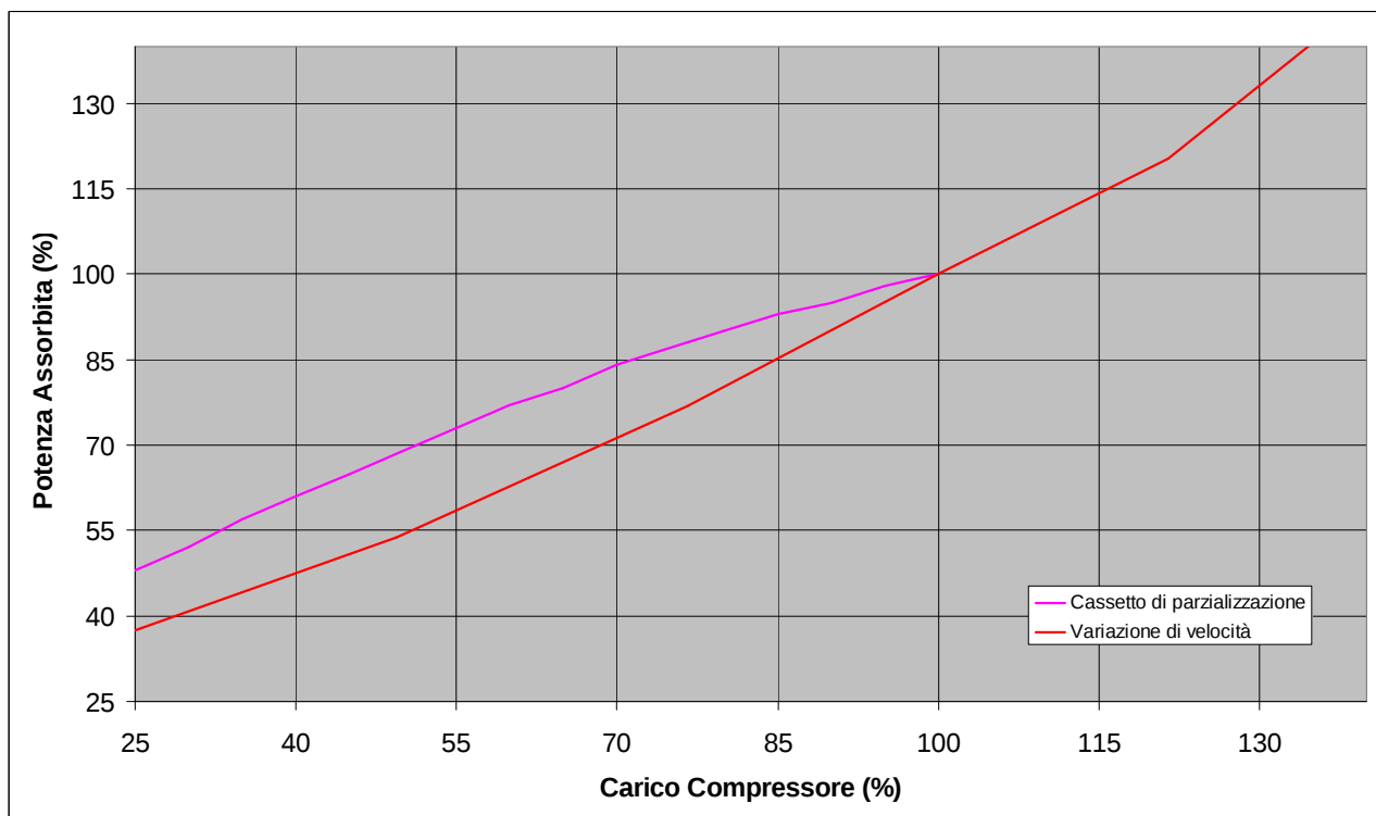
Fig. 15 – Absorción de potencia del compresor en función de la carga
