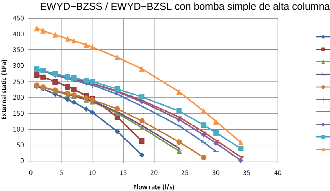
Figura 11 – Kit de bomba de agua de alta columna (optional) - Diagramas presión - caudal
