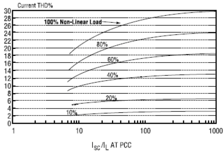
Fig. 19 – Armónica contenido que varía según el porcentaje de cargas no lineales
