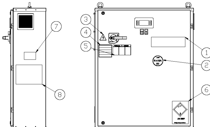
Figura 1 - Identificación de las etiquetas aplicadas al panel eléctrico (Estándar*)
