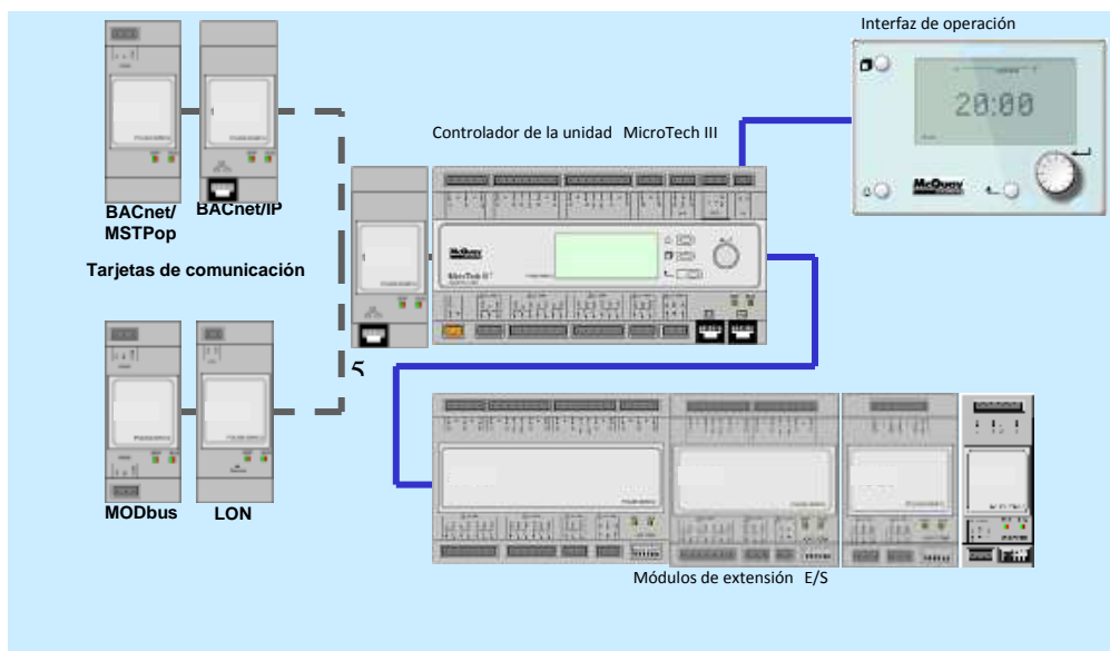
Figura 6: Estructura de hardware
